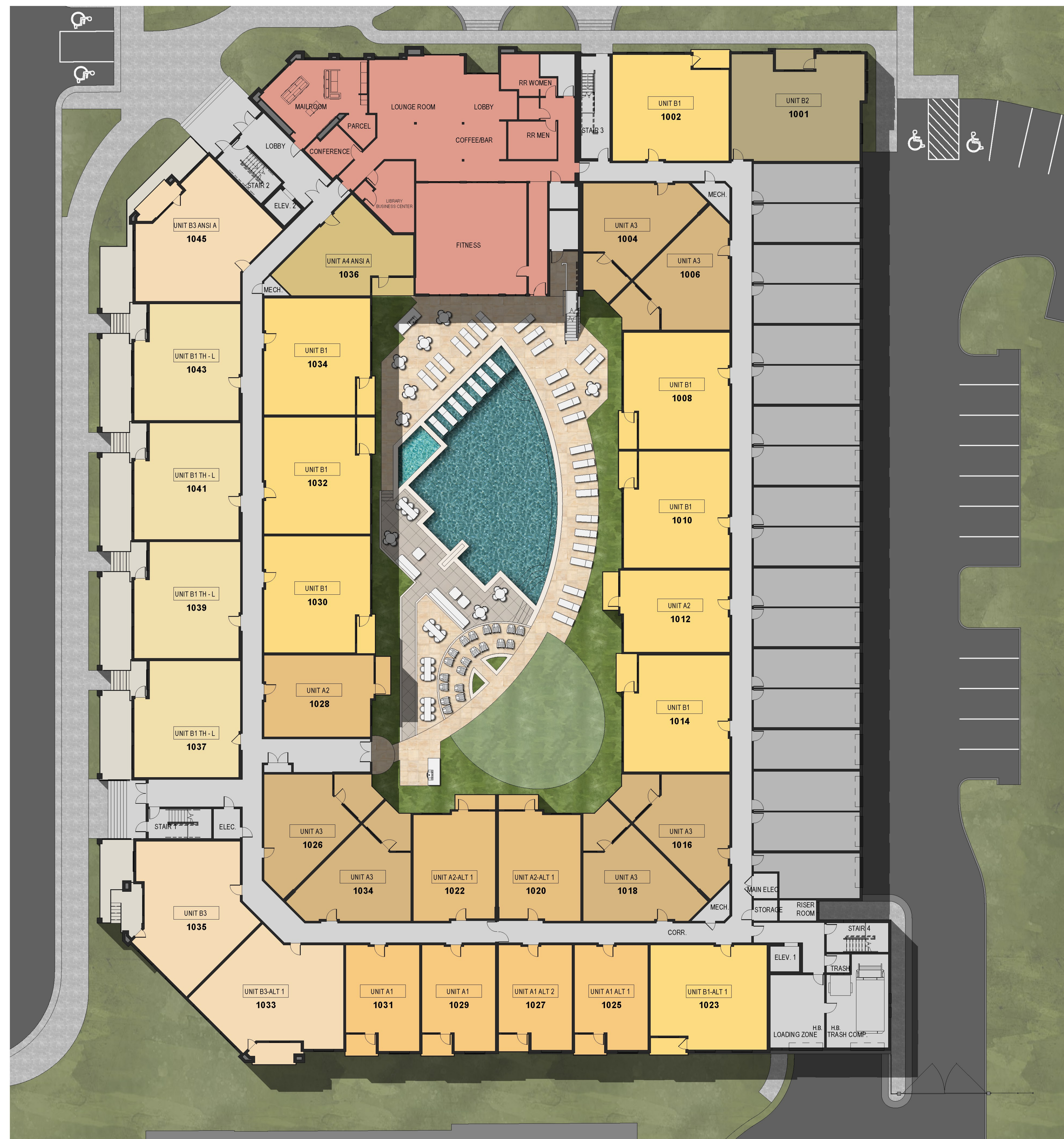
LEVEL 1 SCALE: 1/16" = 1'-0"
